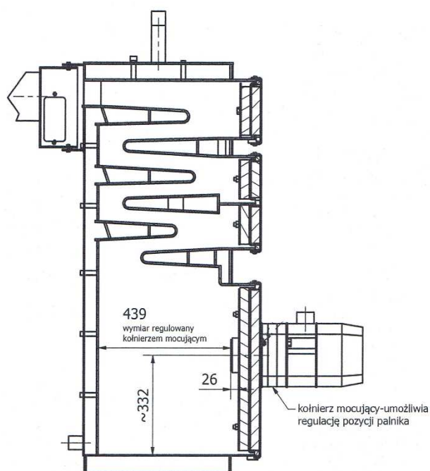
Rys.nr 1. Kocioł Toret 1 ( bez zbiornika paliwa z podajnikiem)
